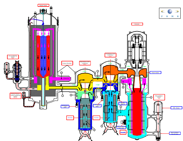
Fig 2. PBMR module
