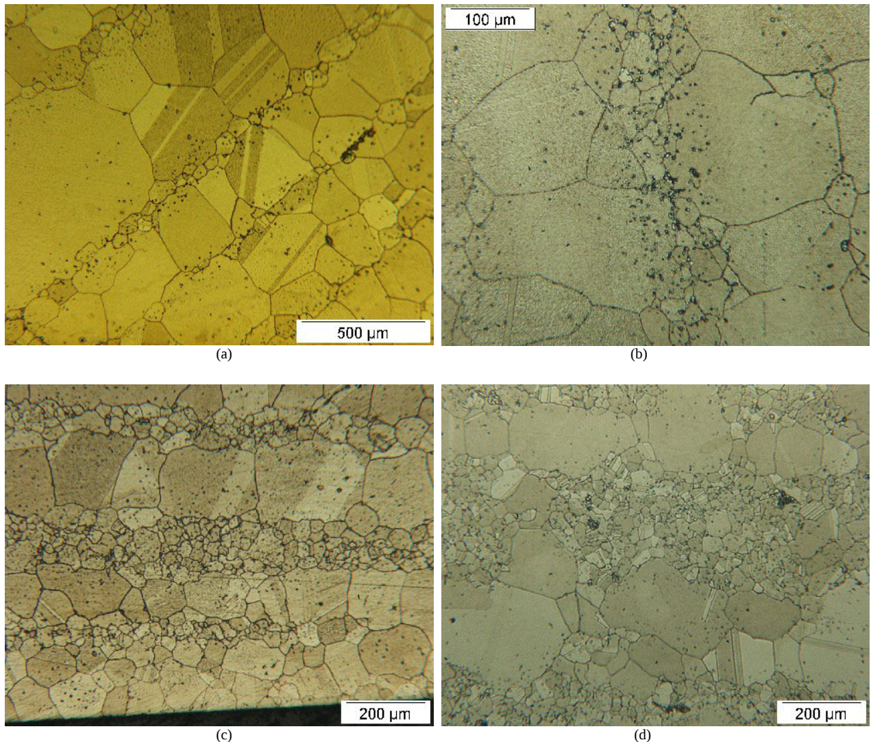
Figures 4 : Microstructural observations of U720 disk. (a) HY1/1 (b) HY1/2 (c) HY1/5 (d) HY1/10.
